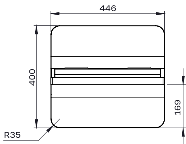
СХЕМА ДИСПЛЕЯ (ВИД СВЕРХУ)
